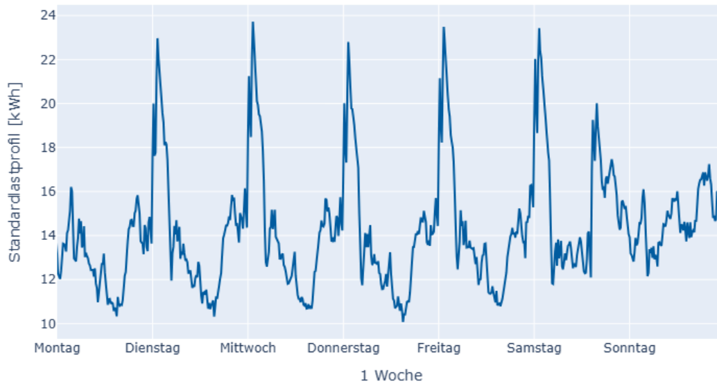
Abbildung 1: Wöchentliches Standardlastprofil als Grundlage für die dynamischen Tarife 2027.
